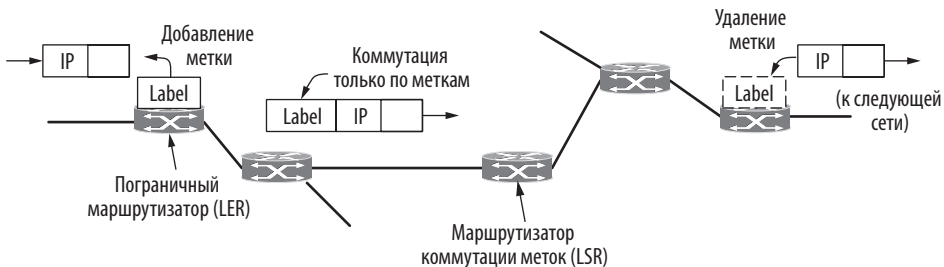
Илл. 5.64. Пересылка IP-пакета через MPLS-сеть
