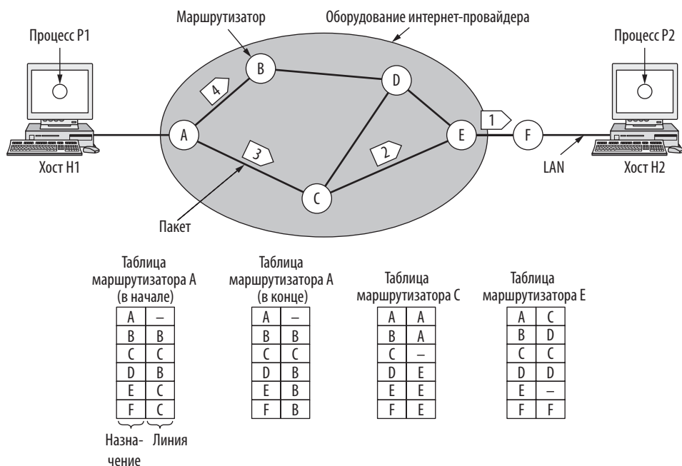
Илл. 5.2. Маршрутизация внутри дейтаграммной сети
