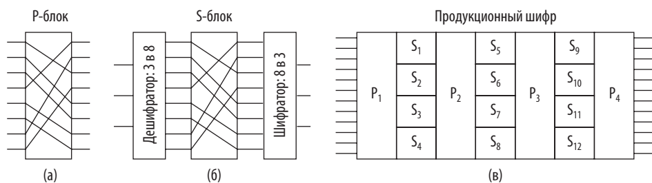
Илл. 8.13. Базовые элементы продукционных шифров: (а) Р-блок; (б) S-блок; (в) продукционный шифр
