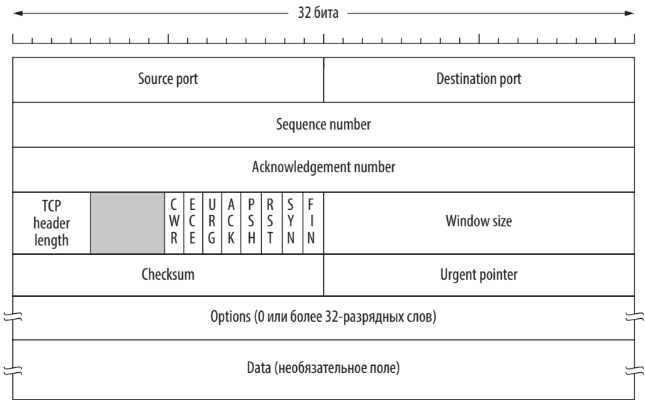
Илл. 6.36. Заголовок ТСП
