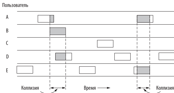
Илл. 4.1. В чистой системе АЛОНА фреймы передаются в абсолютно произвольное время
