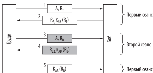
Илл. 8.31. Зеркальная атака
