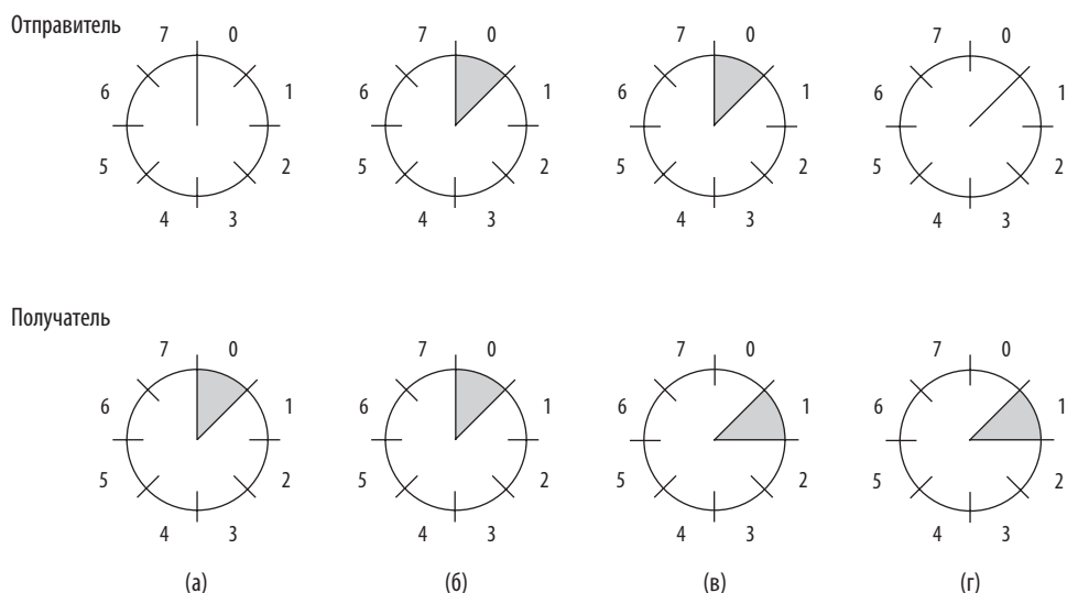
Илл. 3.15. Раздвижное окно размера 1 с 3-битным порядковым номером.
