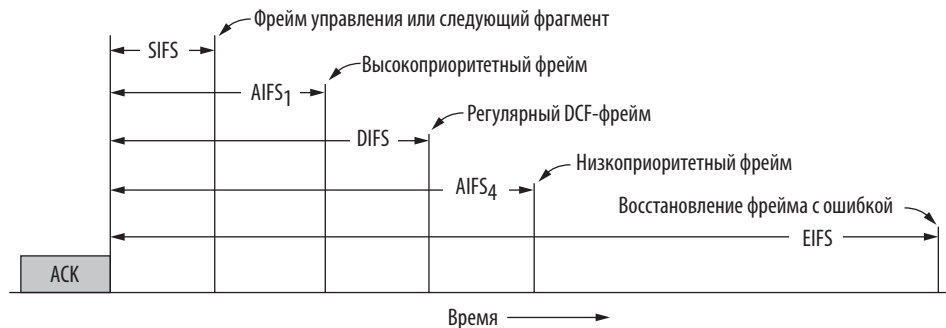
Илл. 4.28. Межфреймовые интервалы в стандарте 802.11
