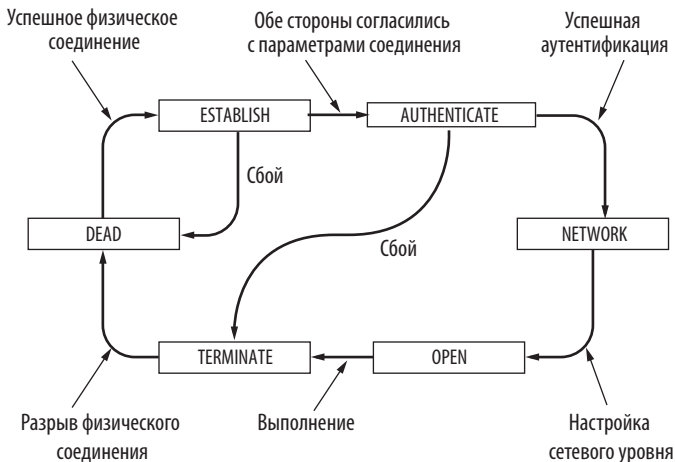
Илл. 3.25. Диаграмма состояний установки и разрыва соединения PPP
