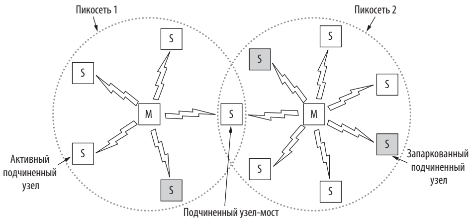
Илл. 4.30. Две пикосети могут объединиться в рассеянную сеть
