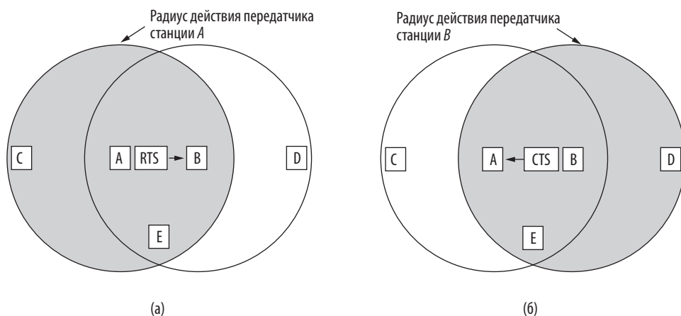
Илл. 4.12. Протокол MACA. (а) Станция А посылает фрейм RTS станции В. (б) станция В отвечает фреймом CTS станции А
