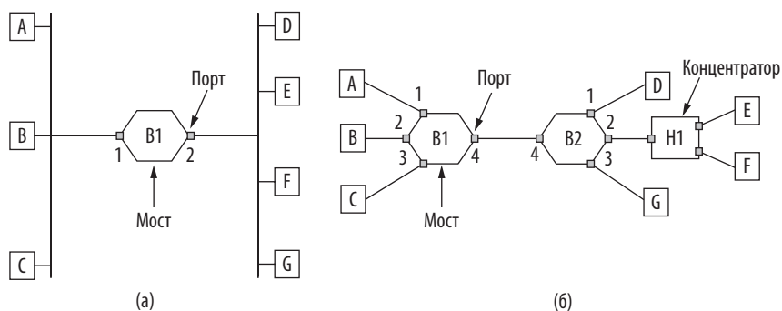
Илл. 4.33. Мосты. (а) Мост, соединяющий две многоточечные LAN. (б) Мосты (и концентратор), соединяющие семь станций по двухточечной схеме
