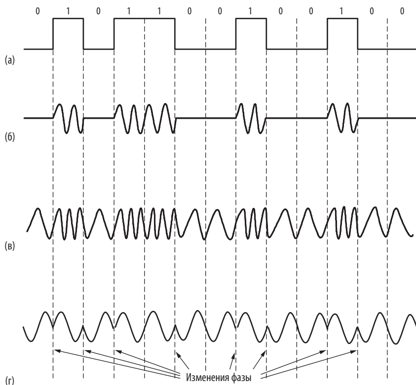
Илл. 2.16. (а) Бинарный сигнал. (б) Кодирование со сдвигом амплитуды. (в) Кодирование со сдвигом частоты. (г) Кодирование со сдвигом фазы
