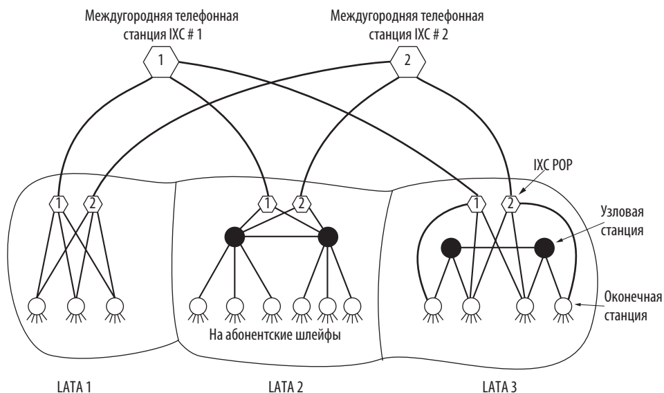
Илл. 2.54. Взаимосвязи LATA, LEC и IXC. Все круги представляют собой коммутаторы LEC, а шестиугольники относятся к IXC с соответствующим номером
