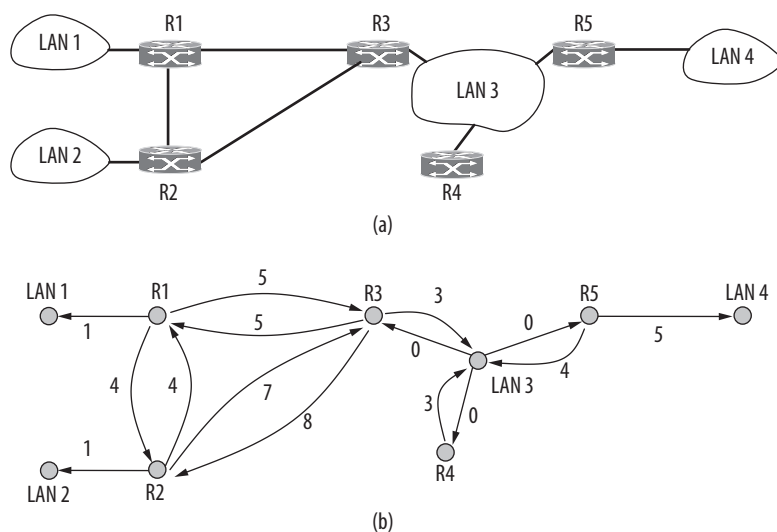
Илл. 5.65. Сеть множественного доступа. (а) Автономная система. (б) Представление (а) в виде графа
