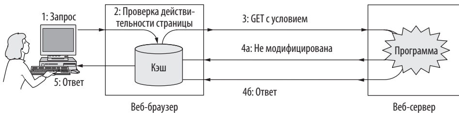
Илл. 7.28. Кэширование HTTP
