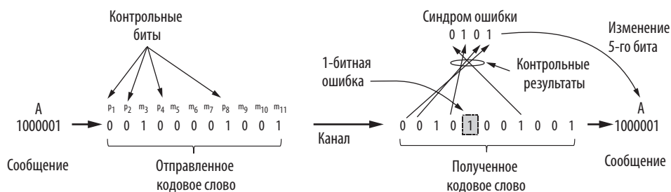
Илл. 3.6. Пример кода Хэмминга (11, 7), исправляющего однобитную ошибку
