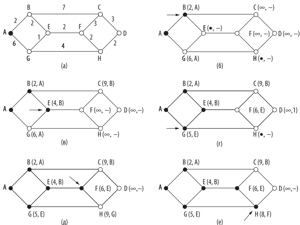
Илл. 5.7. Первые шесть шагов вычисления кратчайшего пути от A к D. Стрелка указывает на рабочий узел
