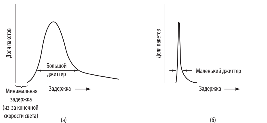
Илл. 6.33. Джиттер: (а) большой; (б) маленький
