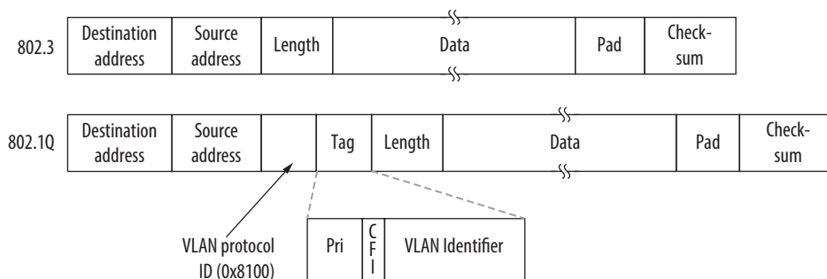
Илл. 4.41. Форматы фреймов Ethernet-стандартов 802.3 (устарел) и 802.1Q
