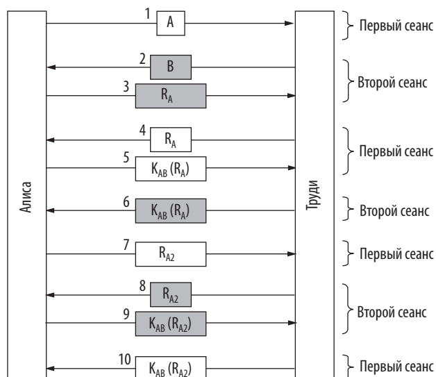
Илл. 8.32. Зеркальная атака протокола, показанного на илл. 8.29
