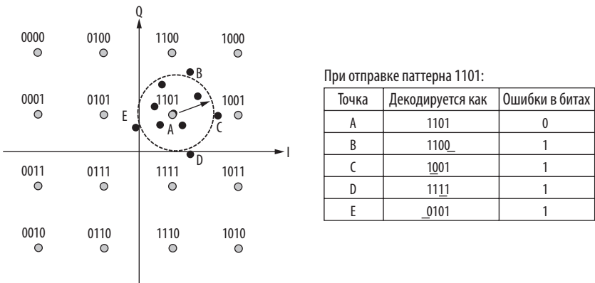
Илл. 2.18. QAM-16, закодированная кодом Грея
