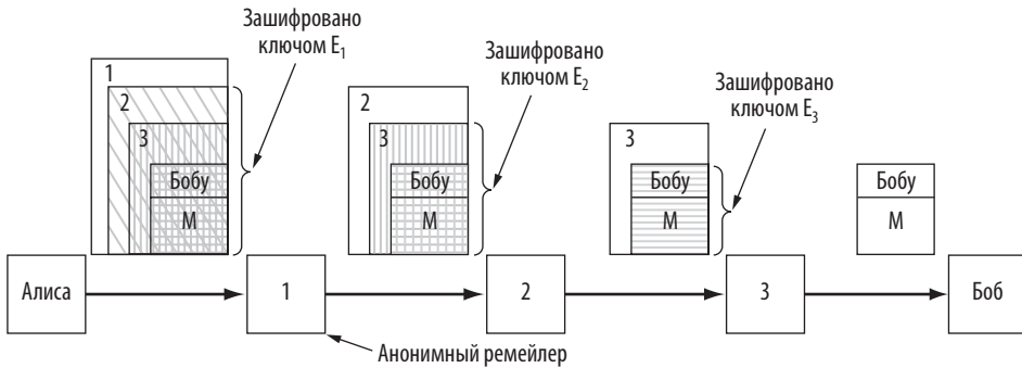
Илл. 8.51. Использование трех анонимных ремейлеров для передачи письма Алисы Бобу
