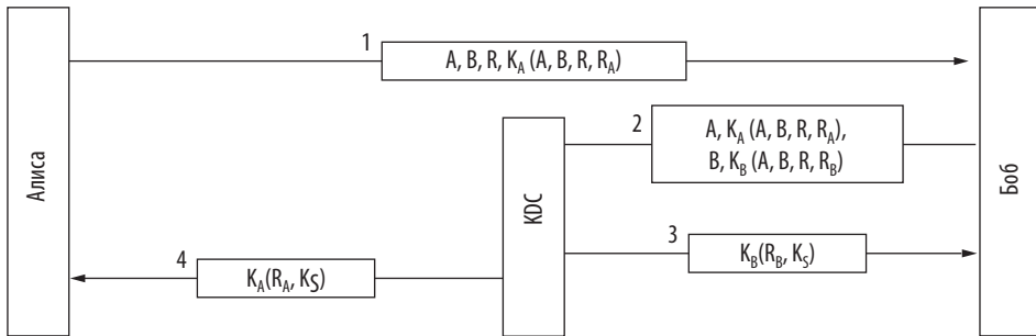
Илл. 8.38. Протокол аутентификации Отуэя — Риса (в слегка упрощенном виде)
