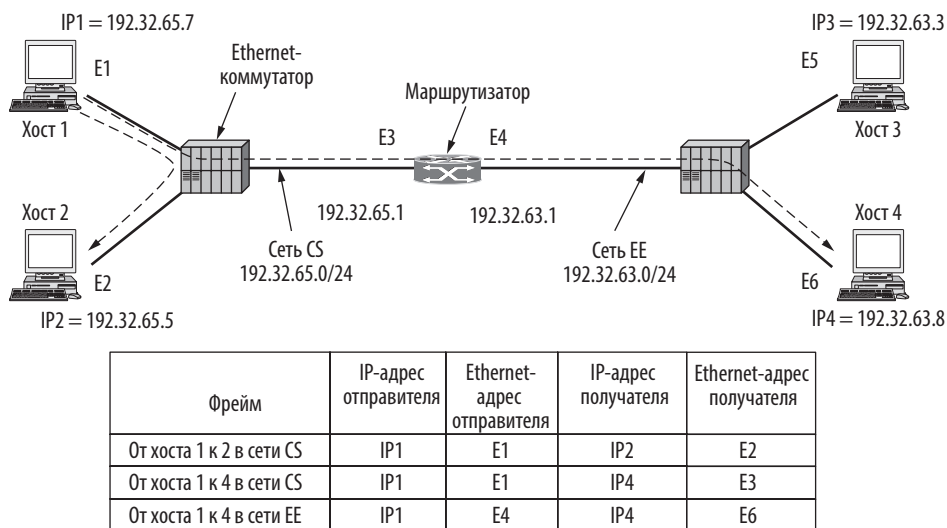
Илл. 5.62. Две коммутируемые LAN Ethernet, соединенные маршрутизатором
