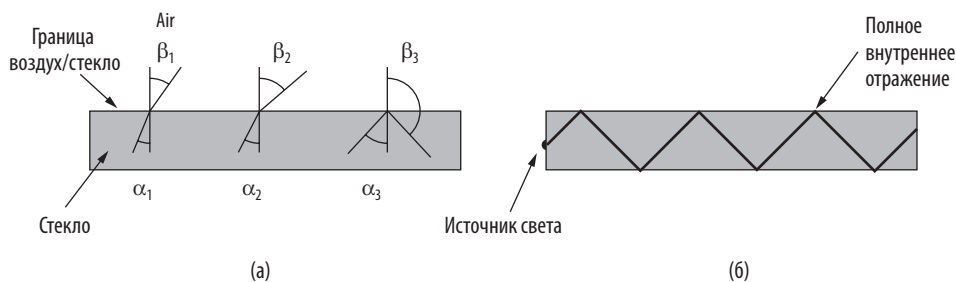
Илл. 2.4. (а) Три примера попадания луча света изнутри кварцевого волокна на границу воздух/стекло под разными углами. (б) Свет, удерживаемый внутри вследствие полного внутреннего отражения
