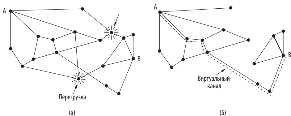
Илл. 5.22. (а) Перегруженная сеть. (б) Участок сети без перегрузки. Также показан виртуальный канал между A и B
