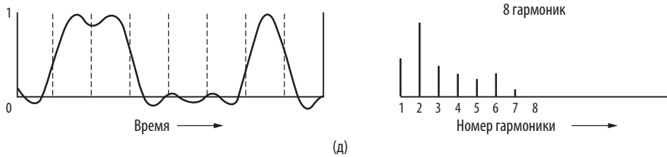
Илл. 2.12. (а) Бинарный сигнал и его среднеквадратичные амплитуды Фурье. (б)–(д) Последовательные аппроксимации исходного сигнала
