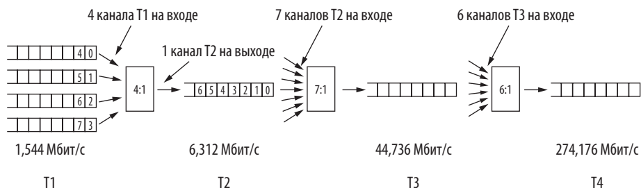
Илл. 2.33. Мультиплексирование каналов T1 в системы связи более высокого порядка
