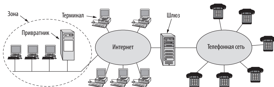
Илл. 7.36. Модель архитектуры Н.323 для интернет-телефонии
