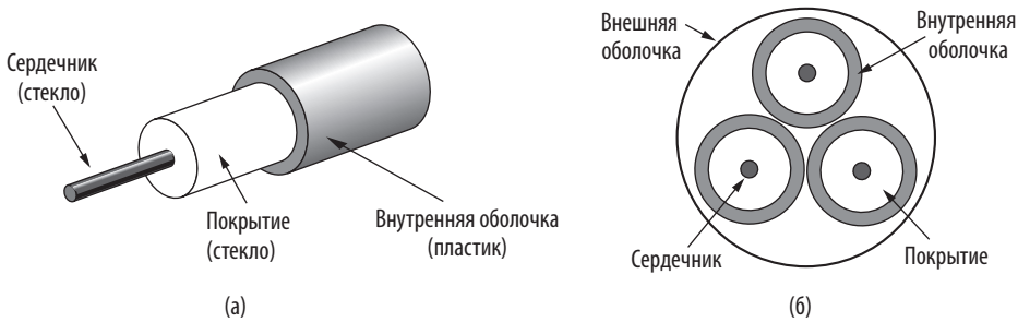
Илл. 2.6. (а) Вид одиночного волокна сбоку. (б) Трехжильный кабель с торца
